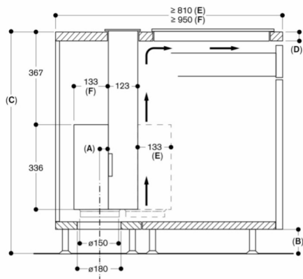
AL 200 с индукционной панелью в двух отдельных вырезках Вид сбоку
