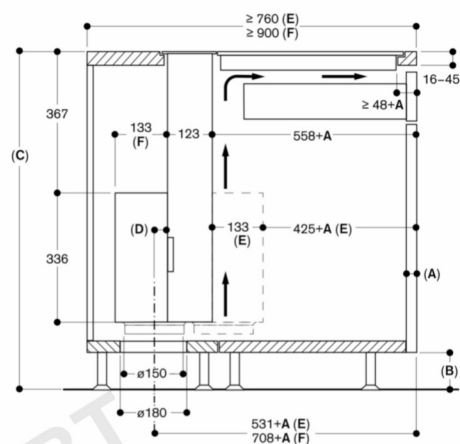
Вид сбоку
